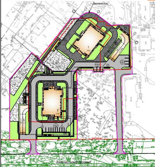
Схема генплана
